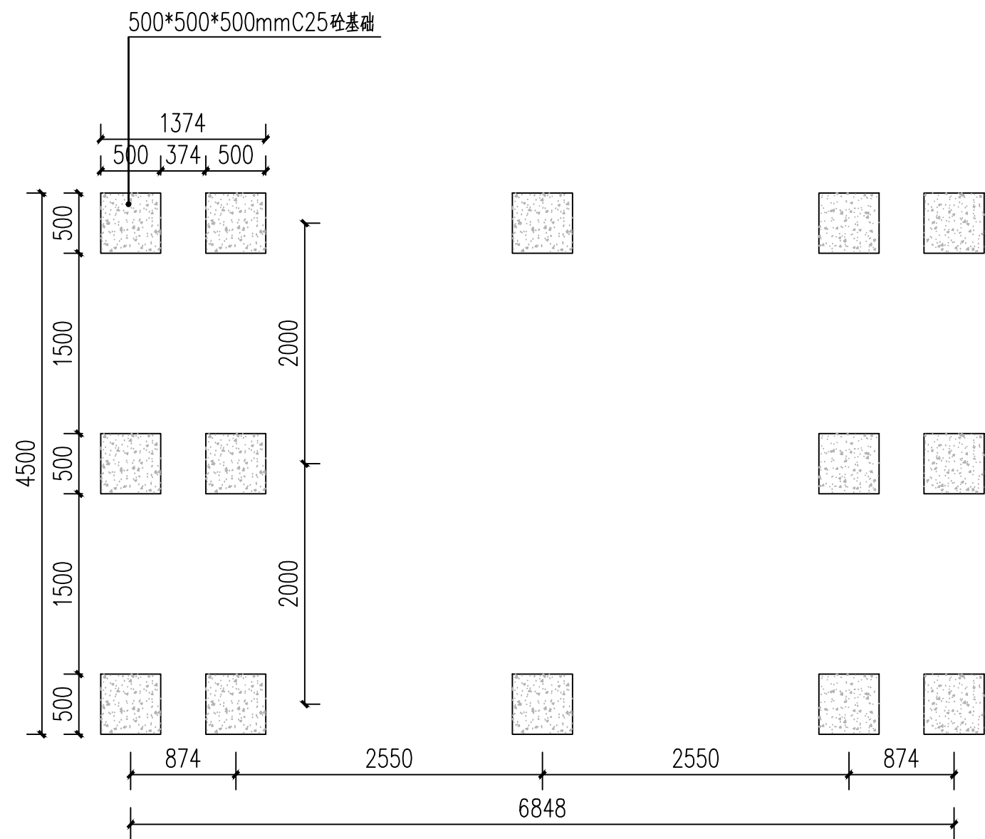
斜绳摆渡示基础平面图
