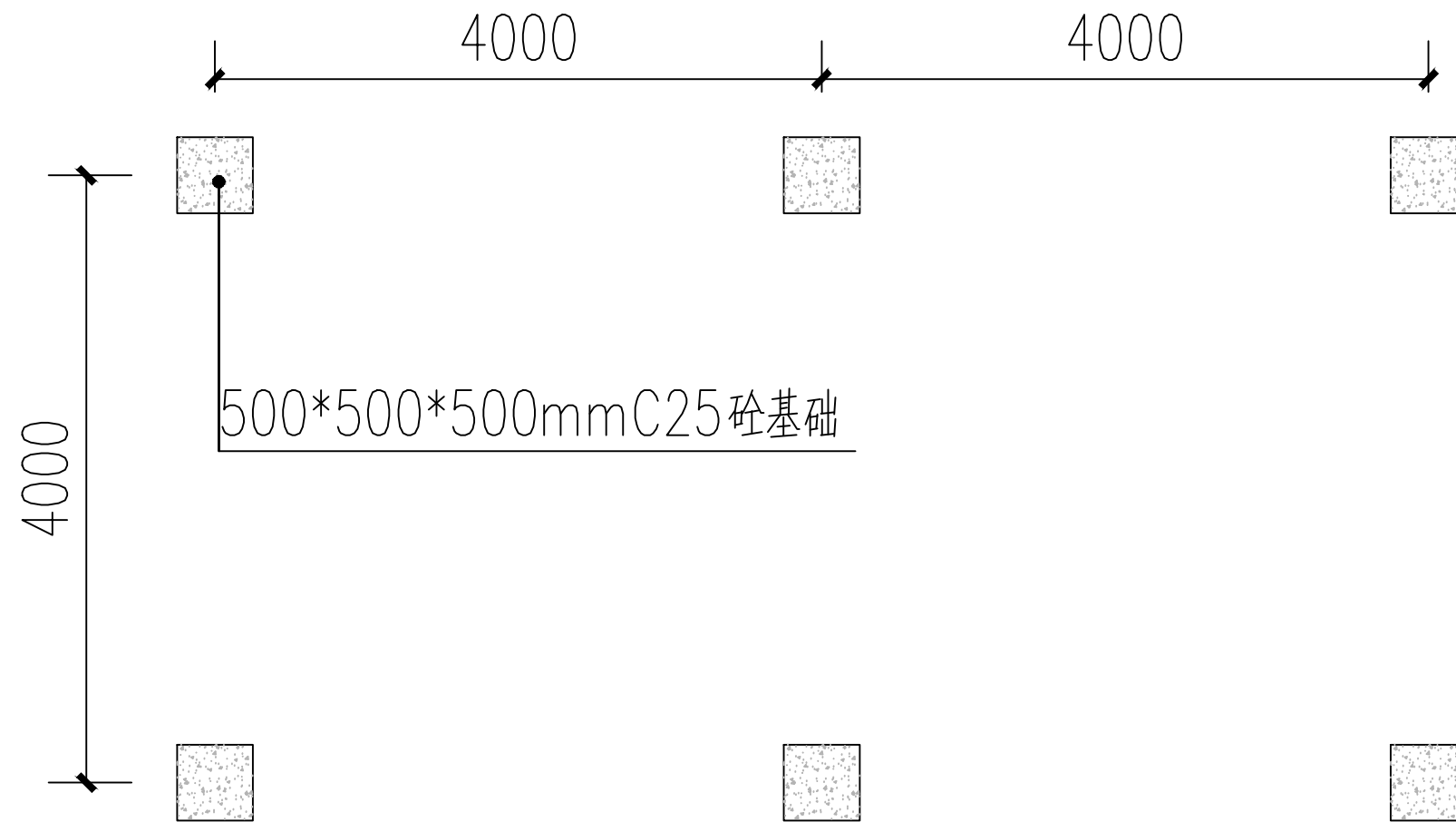
轮胎攀台基础平面布置图
