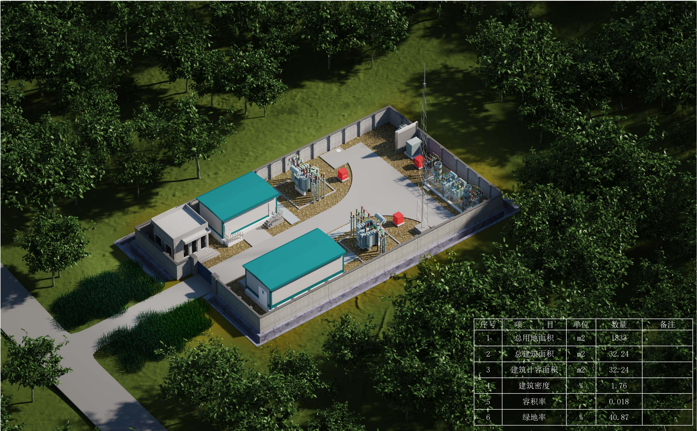
三明宁化河龙 35 千伏输变电工程鸟瞰示意图
